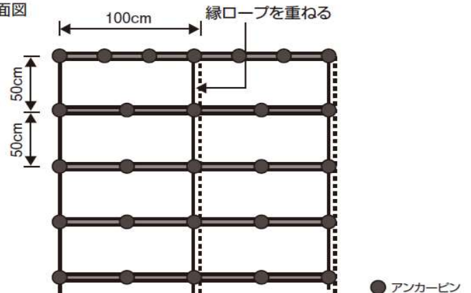
平面図
