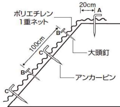
断面図
